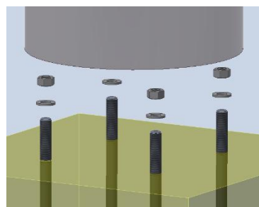
Type B : Scellement intérieur borne
