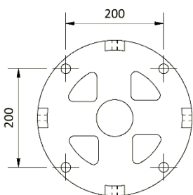
Type A : Scellement sur platine amovible
