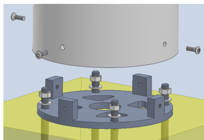
Type A : Scellement sur platine amovible
