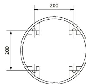
Type B : Scellement intérieur borne
